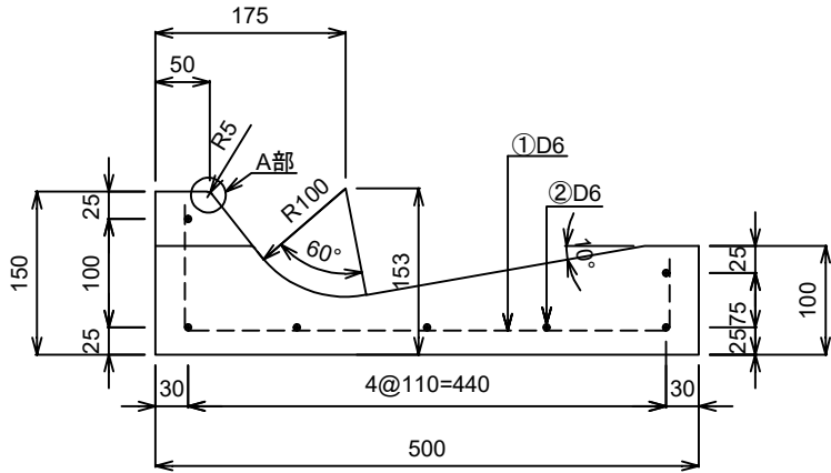
断面図
