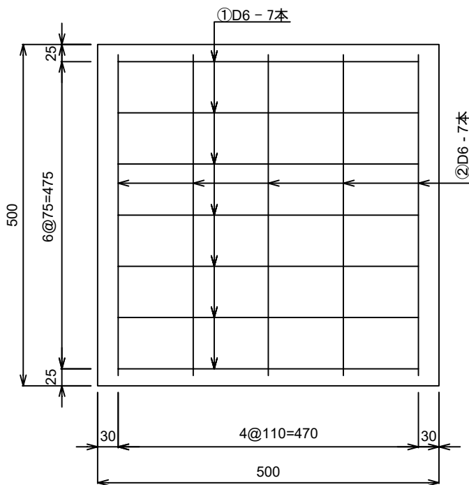
配筋図
