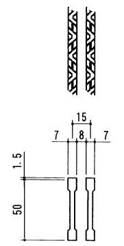
ベアリングバー 詳細図
