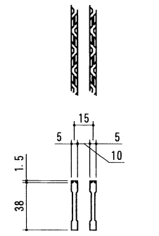
ベアリングバー 詳細図
