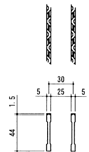
ベアリングバー 詳細図
