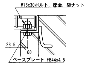
ボルト固定 詳細図
