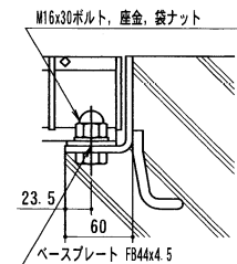
ボルト固定 詳細図
