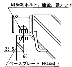
ボルト固定 詳細図
