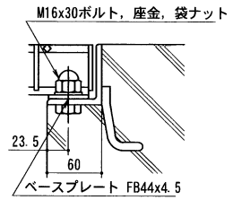
ボルト固定 詳細図
