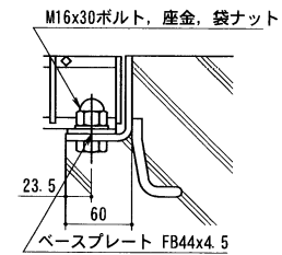
ボルト固定 詳細図
